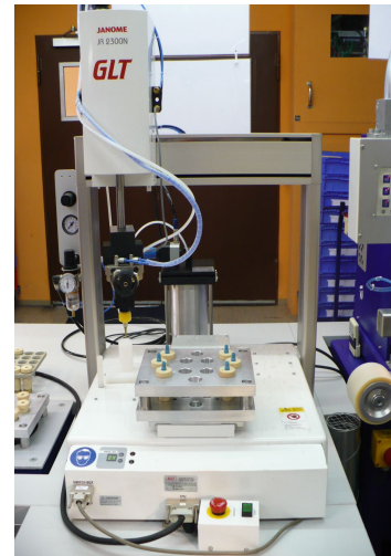
3-Achs-Roboter zum Kittten
